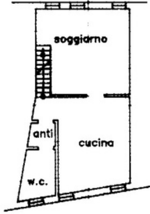
PIANO PRIMO H = 2.40 m.
